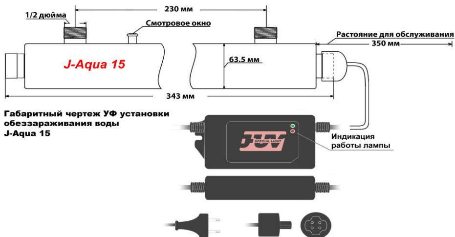
Рисунок 1. Габаритный чертеж J-Aqua 15
